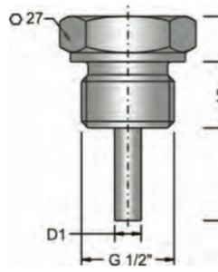
G 1/2" ISO 228-1
